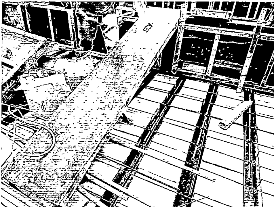
Foto N° 01: Suministro e instalación de las tuberías 1/2" en el techo del edificio de frío
