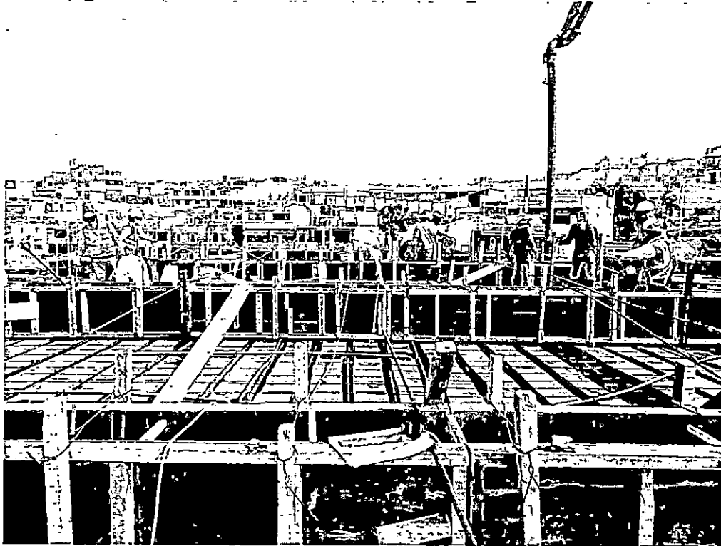
Foto N° 03: Suministro e instalación de las tuberías 2" en el techo del edificio de frio.
